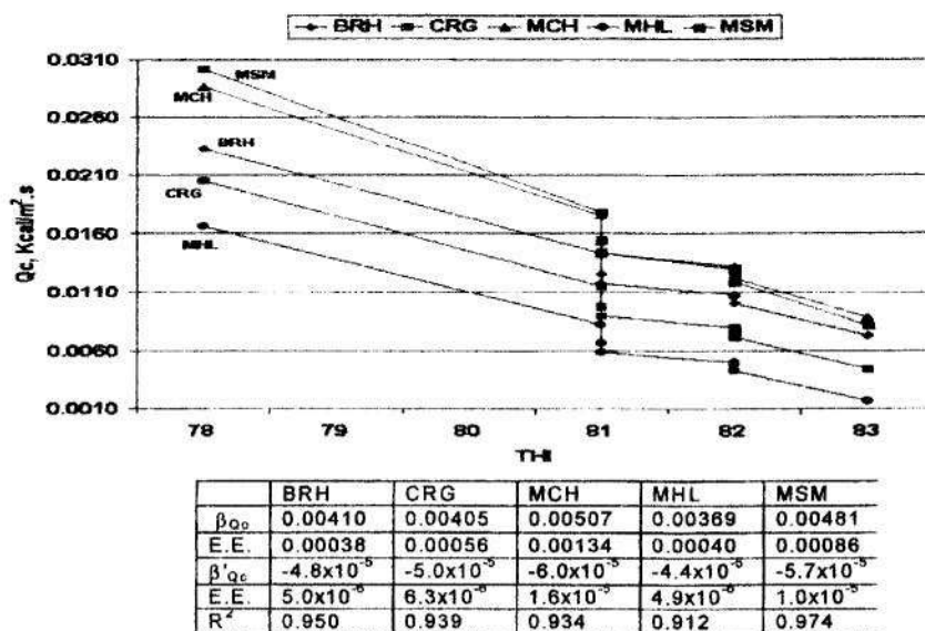
FIGURA 7. CONVECCIÓN CALÓRICA POR GRUPO RACIAL Y THI.
