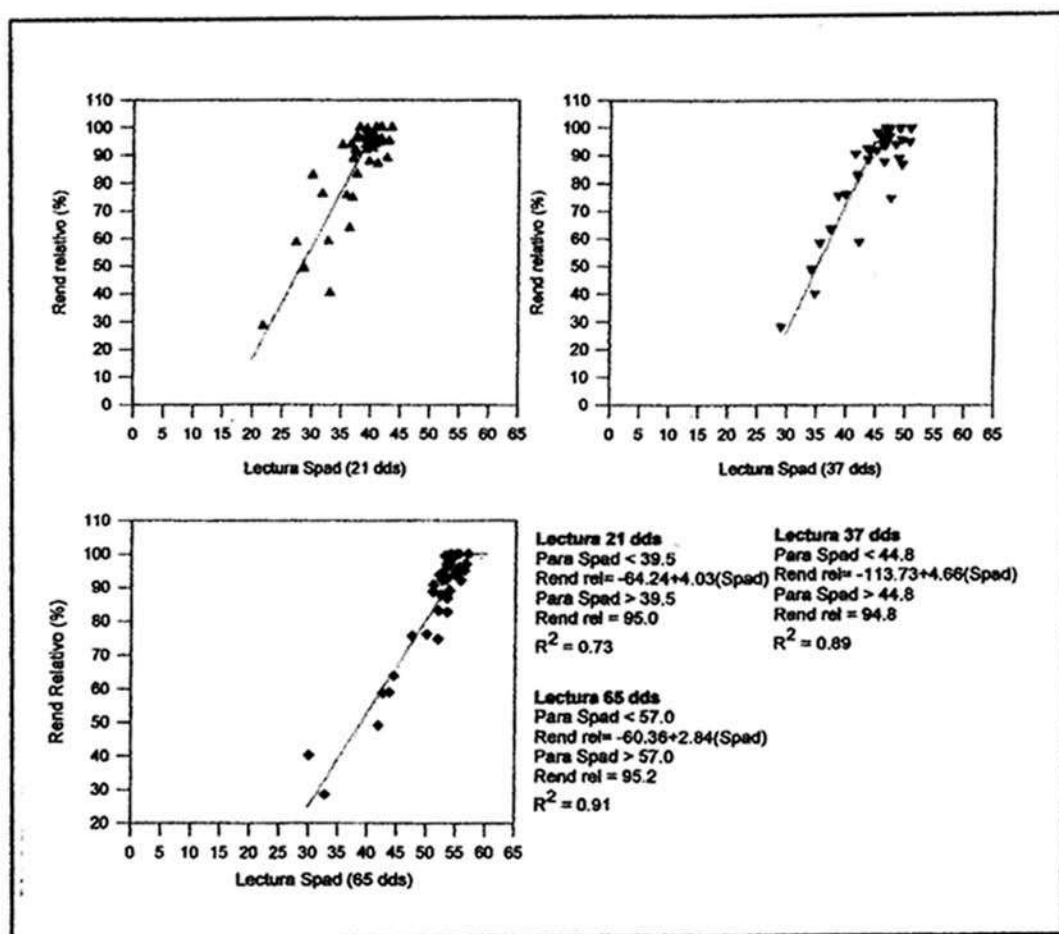
FIGURA 1. ECUACIONES DE LA RELACIÓN DE LA LECTURA DEL SPAD-502 A LOS 21, 37 Y 65 DDS CON EL RENDIMIENTO RELATIVO. AZUERO, PANAMÁ. 2002.
