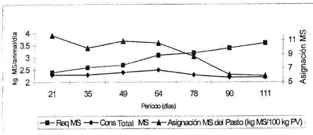
FIGURA 4. REQUERIMIENTO DE MATERIA SECA, CONSUMO TOTAL DE MATERIA SECA Y ASIGNACIÓN DE MS DEL PASTO (kg MS/100 kg PV), TRATAMIENTO 1.
