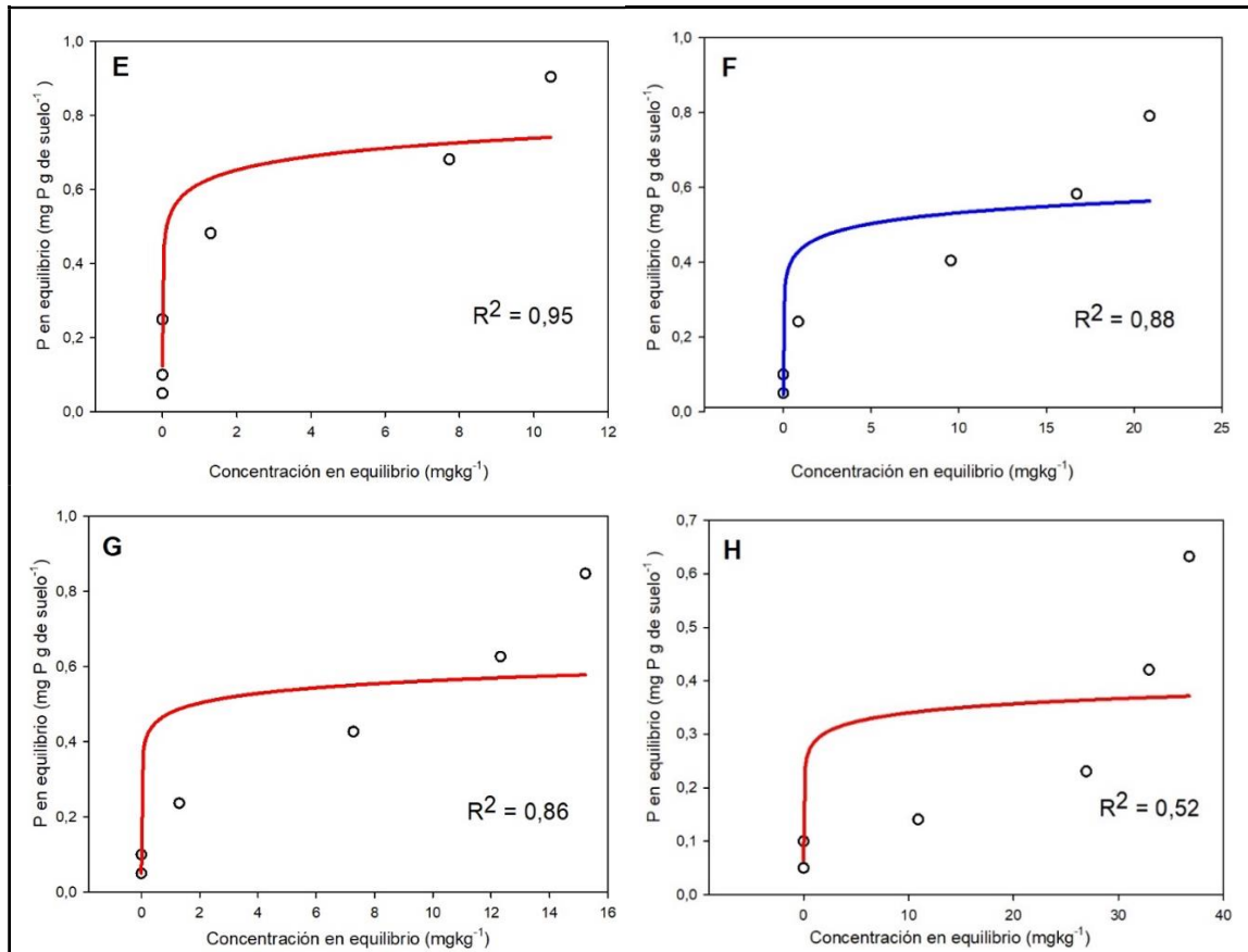
Figura 2. Isotermas de Langmuir para los suelos de las localidades del norte: Guararé (E), El Ejido (F), Llano Abajo (G) y La Colorada (H).
